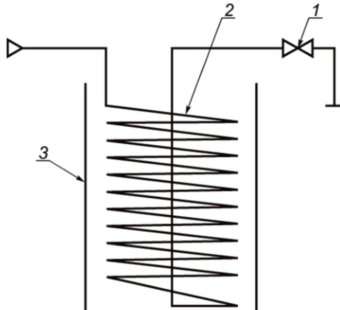
1 - игольчатый вентиль; 2 - змеевик; 3 - сосуд для охлаждающей смеси
